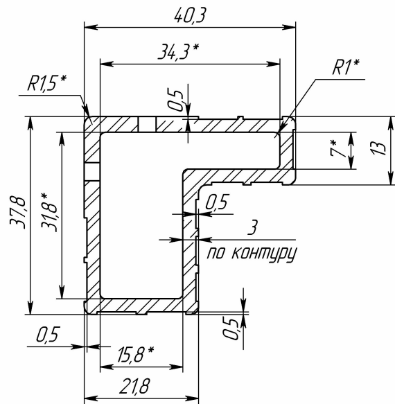
Г-Г (1:1) (1)
