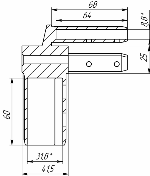
Т-Т (1) 2 места
