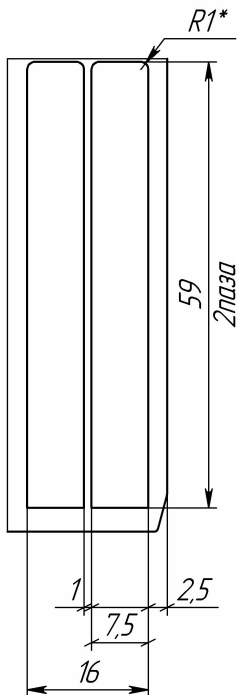
П (1:1) (1) 4 места
