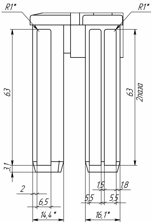
С (1:1) (1) 2 места
