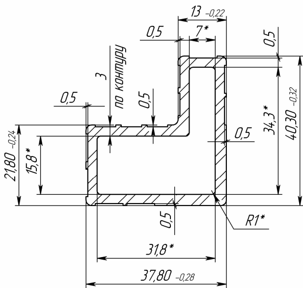
Д-Д (1:1) (1)
