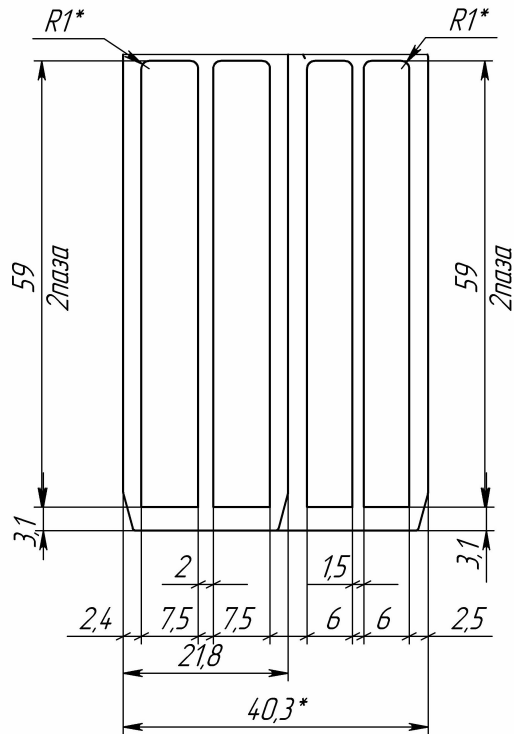
Р (1:1) (1) 2 места
