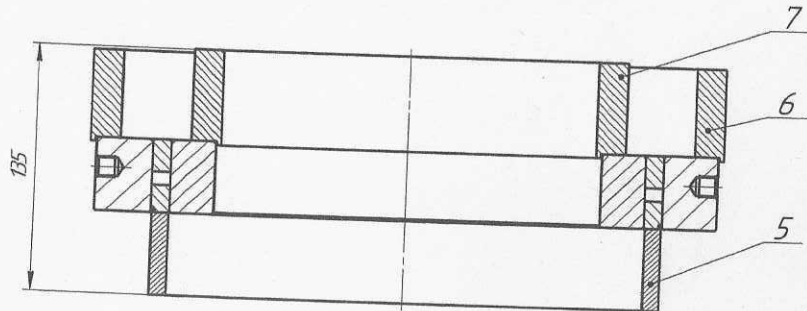
Схема распрессовки (1:2)
