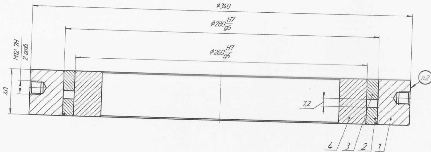
Схема распрессовки (1:2)
